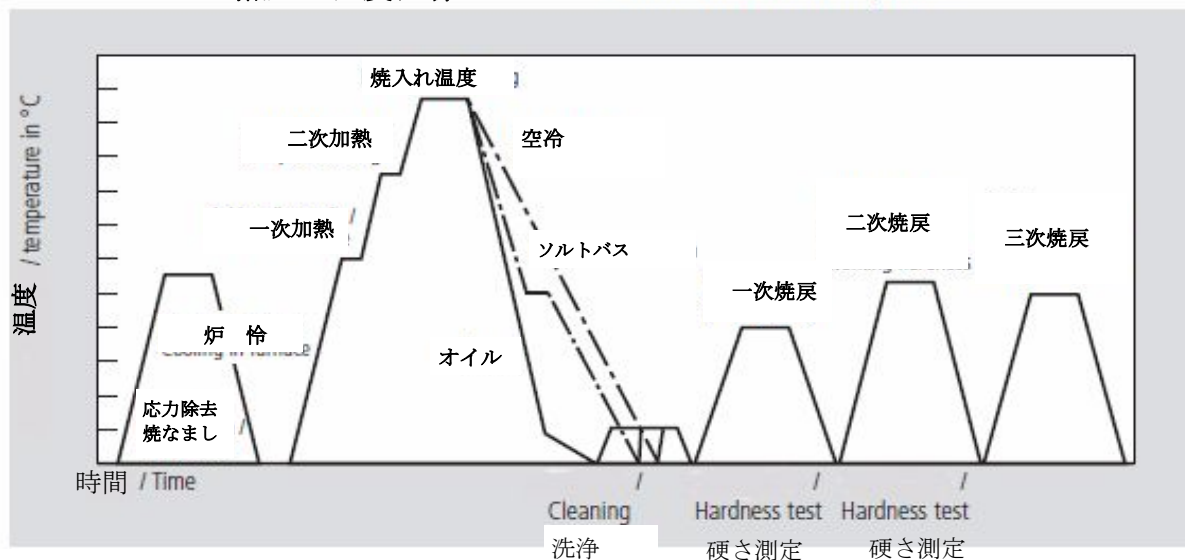
W403の熱処理温度曲線
